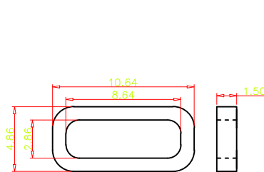
建议的胶圈尺寸
