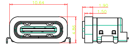
加防水圈示意图
