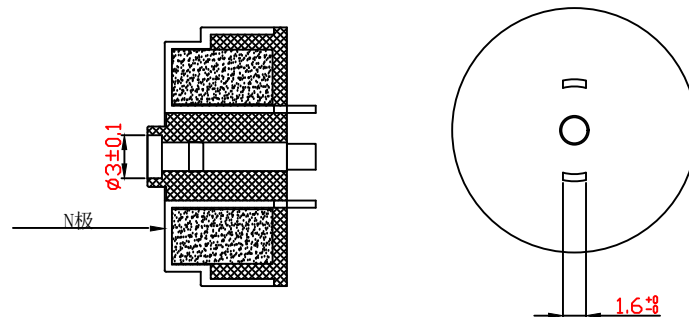
磁吸母头
