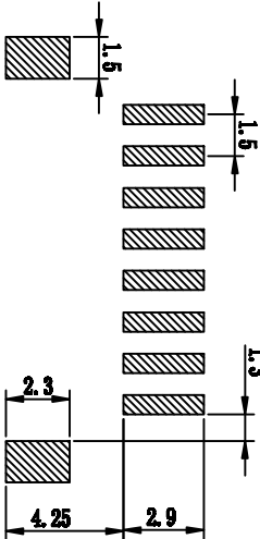
印制线路板 (公差±0.05)
